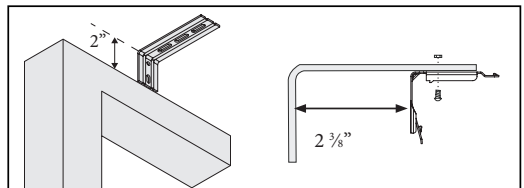
Installation extérieur-cadre avec supports d'extension Surface de 2 po minimum
