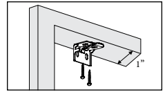
Installation peu profonde : Surface de 1 po minimum Installation à plat : Surface de 3 3/4 po minimum
